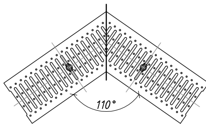
Стыковка лотков
