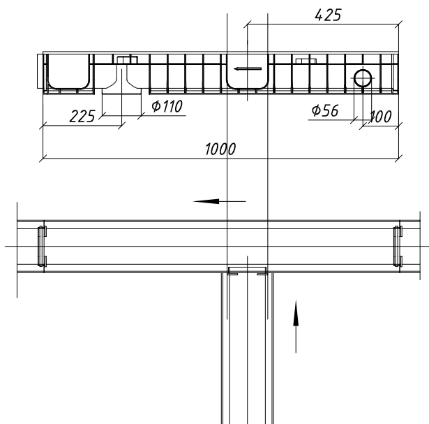
"Т" образный стык лотков
