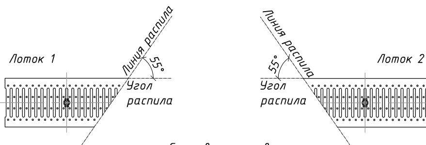
Стыковка лотков
