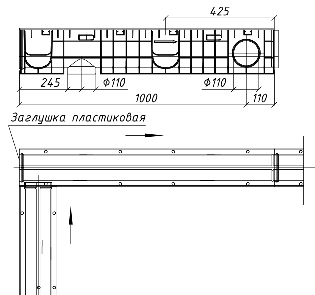
"Г" образный стык лотков
